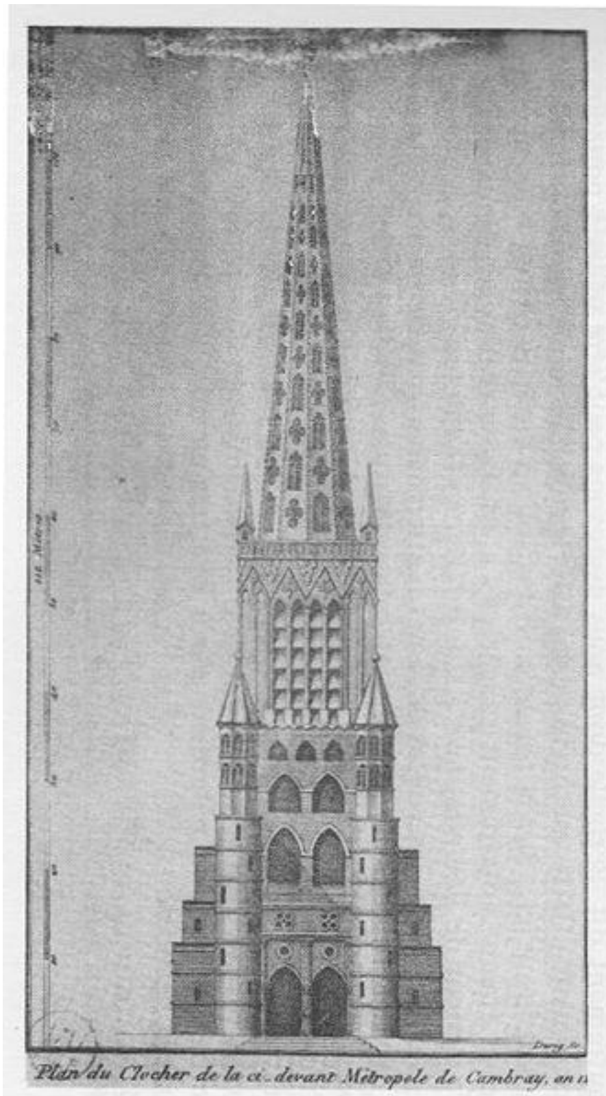
Clocher de la cathédrale dessiné par Amédée Boileux, avec la légende : « Plan du Clocher de la ci-devant Métropole de Cambrai, an 12 »
